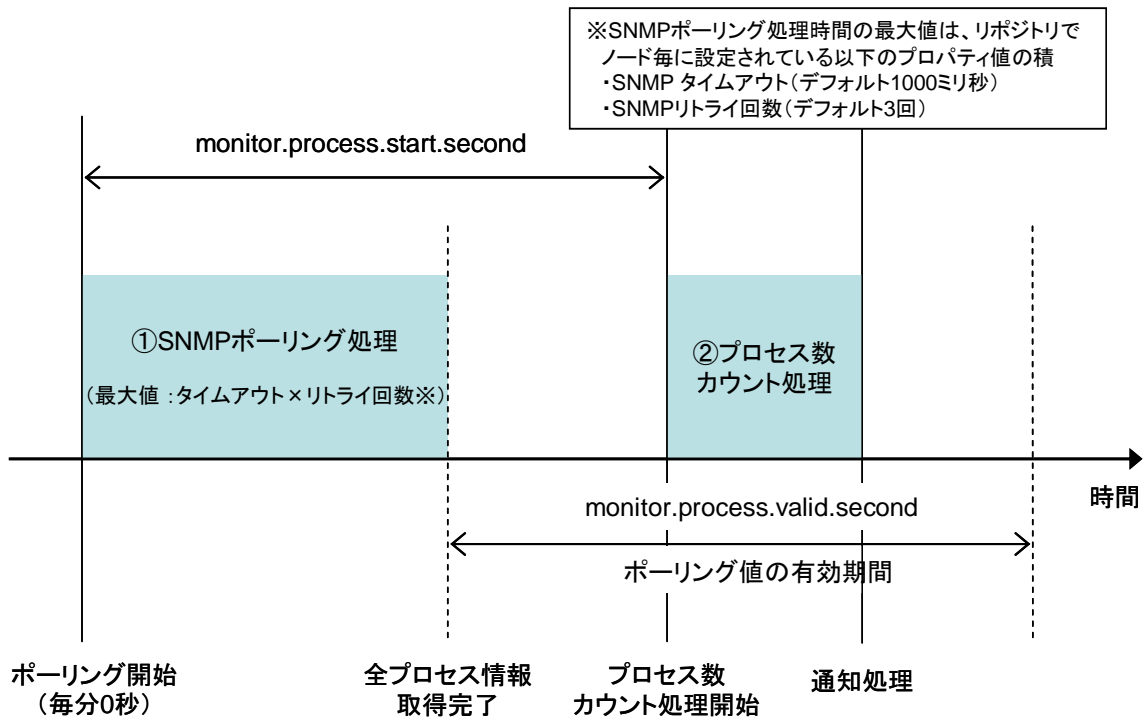
図 1 プロセス監視の処理
